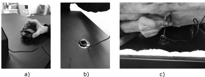
Figure 8 - Mise en place de la sonde de température
