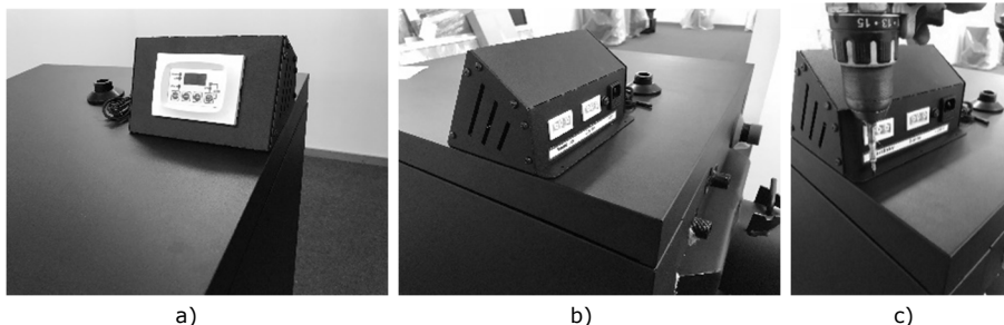
Figure 7 - Placement du contrôleur de ventilateur
