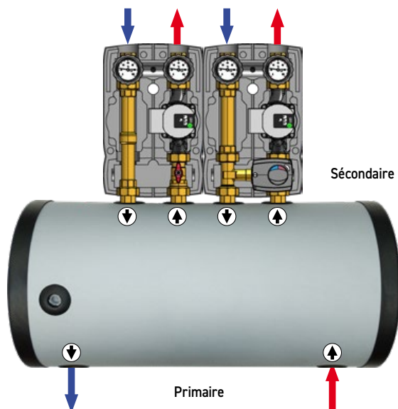
Schéma d'application: bouteille montage horizontal
